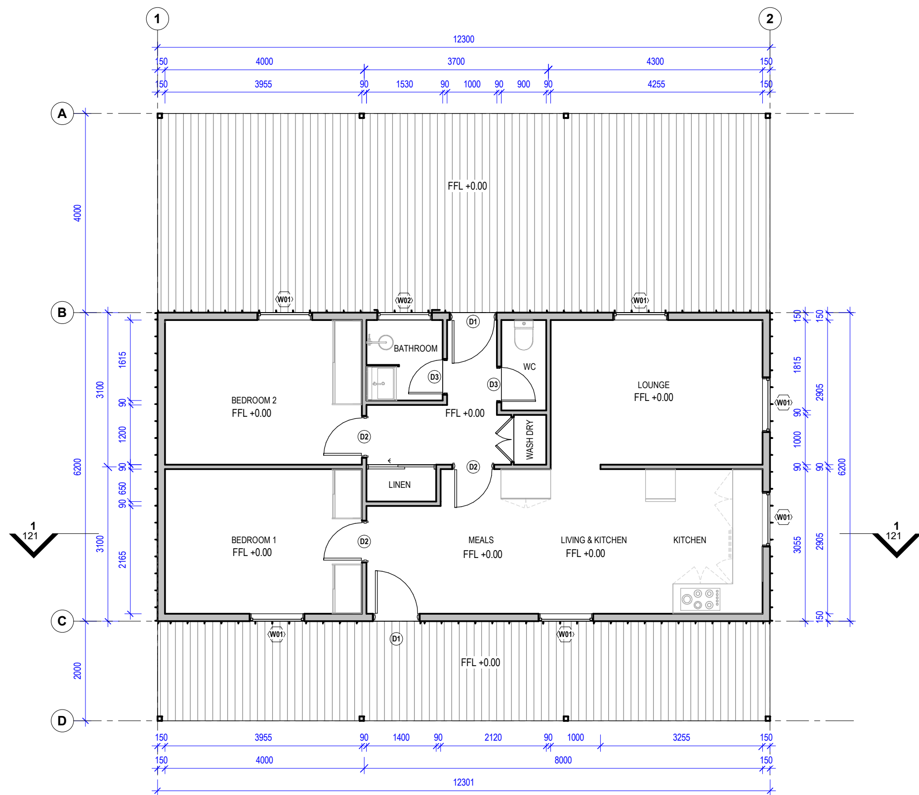
1 FLOOR PLAN 1 : 75
